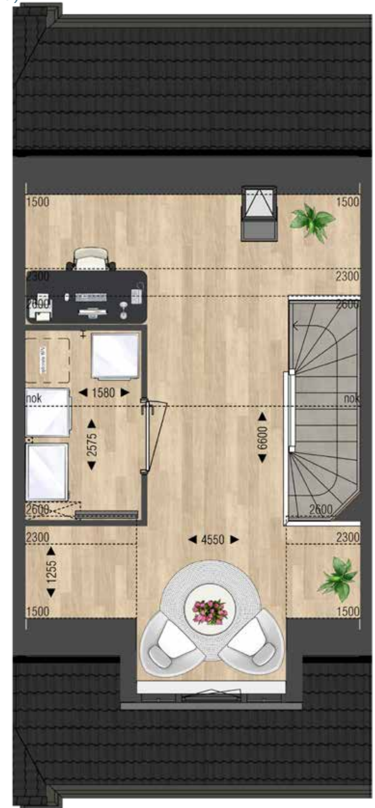
Tweede verdieping
